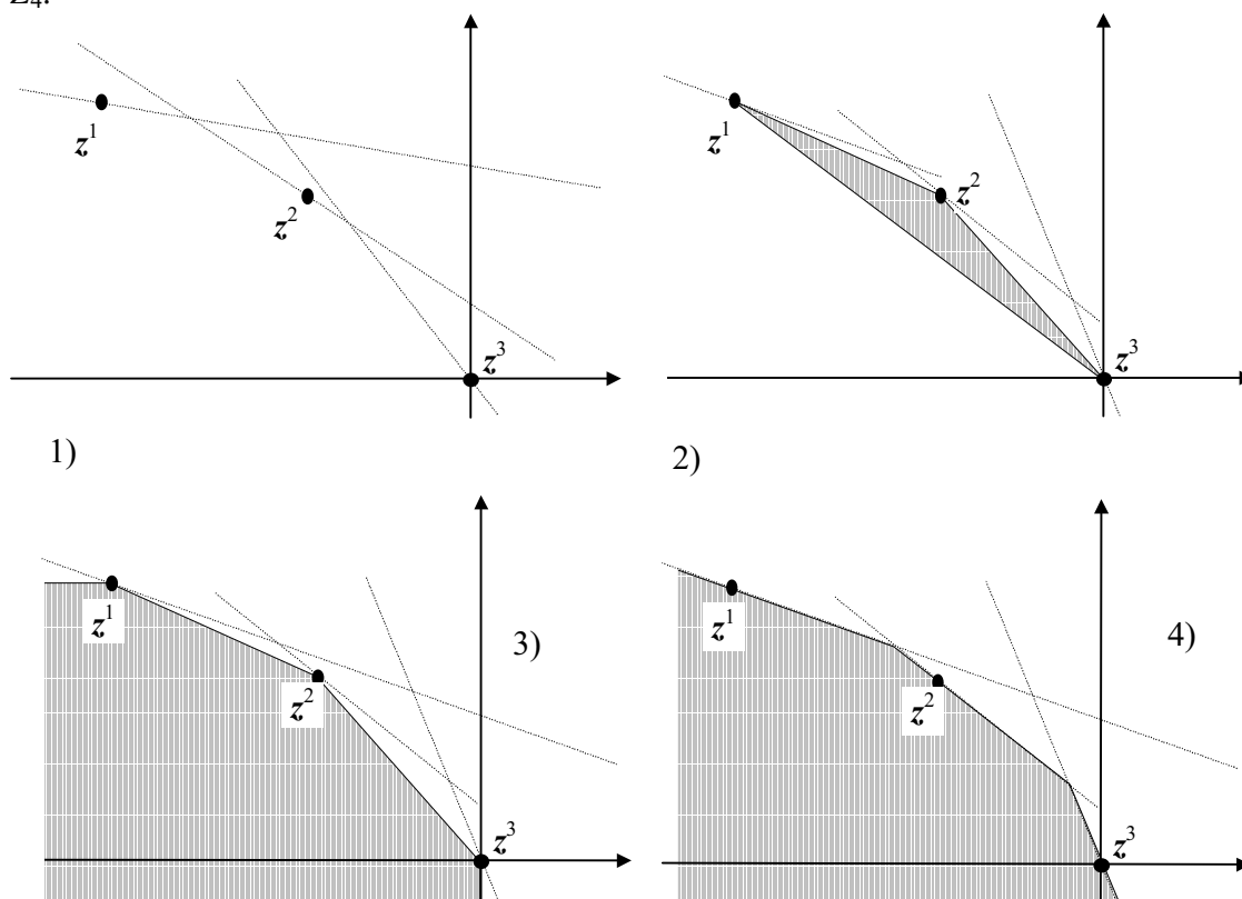
Рисунок 7. Возможные способы восстановления множества Z по наблюдаемым точкам
